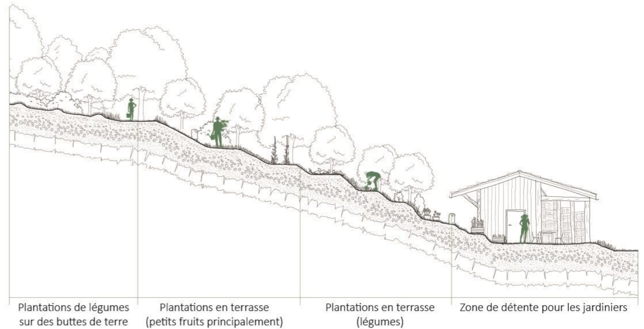
Coupe AA'
